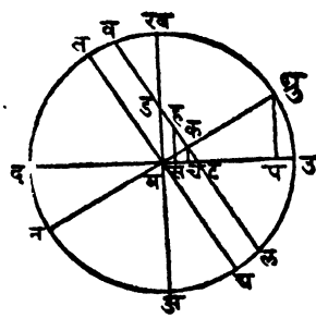
अक्षक्षेत्रे दाखविणारी आकृति.
